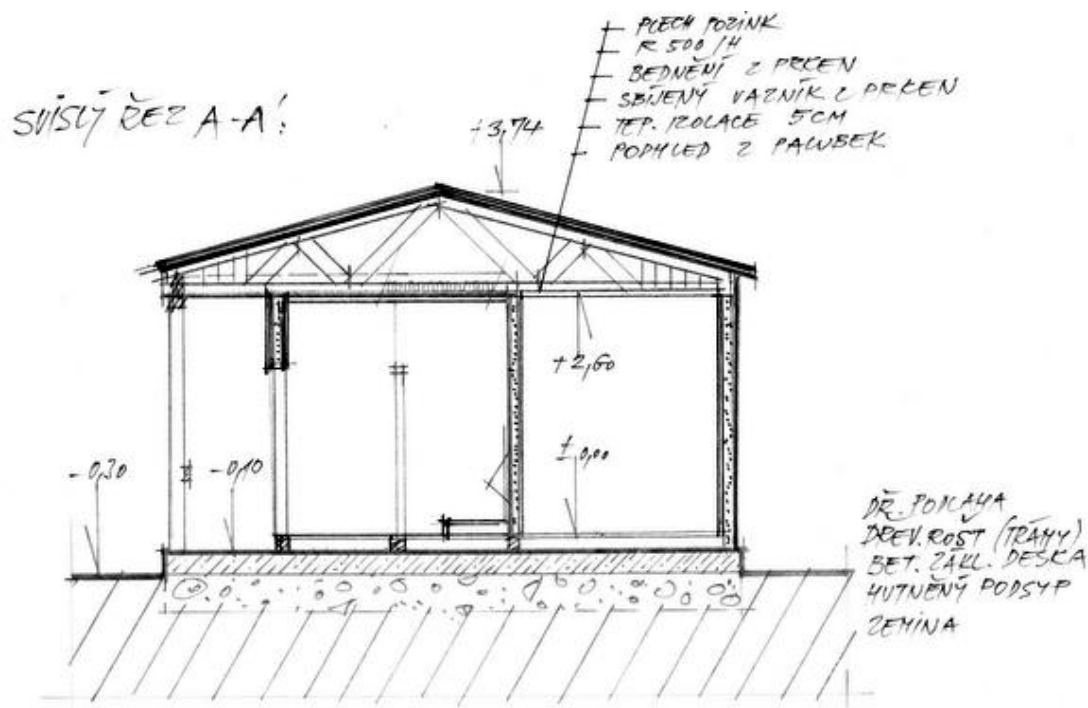
Obr. č. 31: jeden z řezů stavebním objektem sociálního zařízení z dokumentace pro stavební povolení
